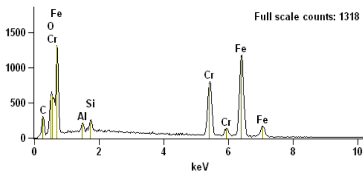
Fig. 7. Análise de EDS CP2C. Fonte: Senai.
