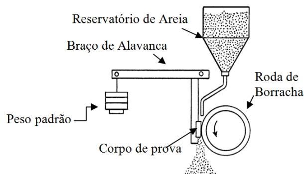
Fig. 2. Esquema de funcionamento do equipamento de ensaio abrasômetro. Adaptado de ASTM G65-04, 2010.
