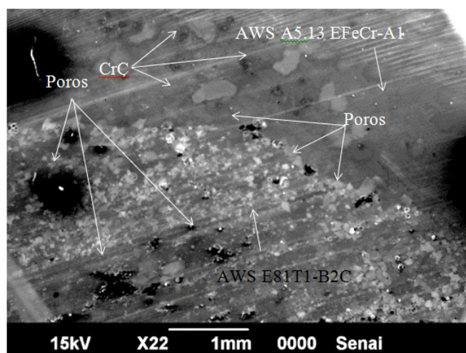
Fig. 8. MEV CP3A. Fonte: Senai.
