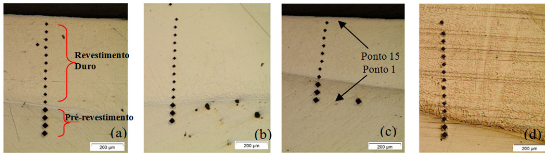
Fig. 3. Perfil de microdureza. (a) CP2A; (b) CP3A; (c) CP4A; (d) CP5A.
