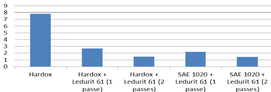
Fig. 5. Taxa de desgaste abrasivo ( \text{mm}^3/\text{m} \times 10^{-3} ).
