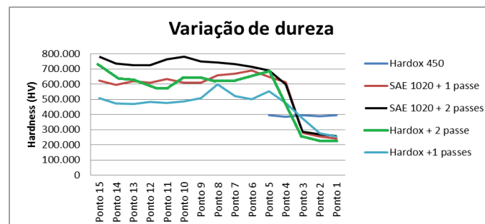
Fig. 4. Análise de microdureza (HV).
