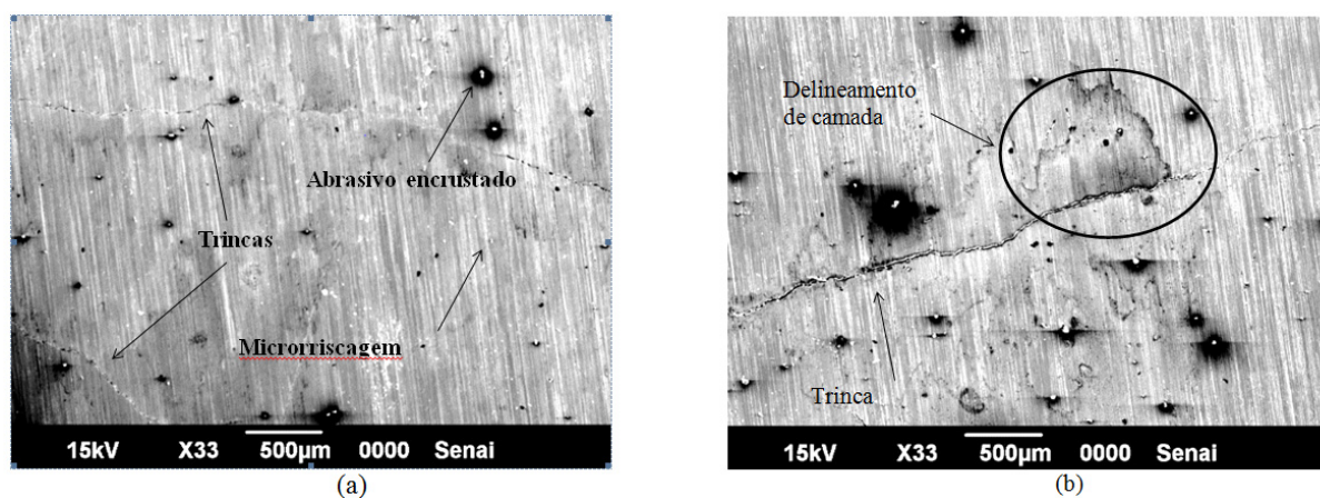
Fig. 6. A análise MEV a) da face desgastada CP2C (Hardox +1 passe), b) da face desgastada CP4C(SAE 1020 +1 passe).
